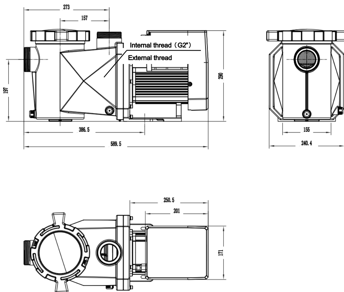
Figur 1 – Pumpens mått
